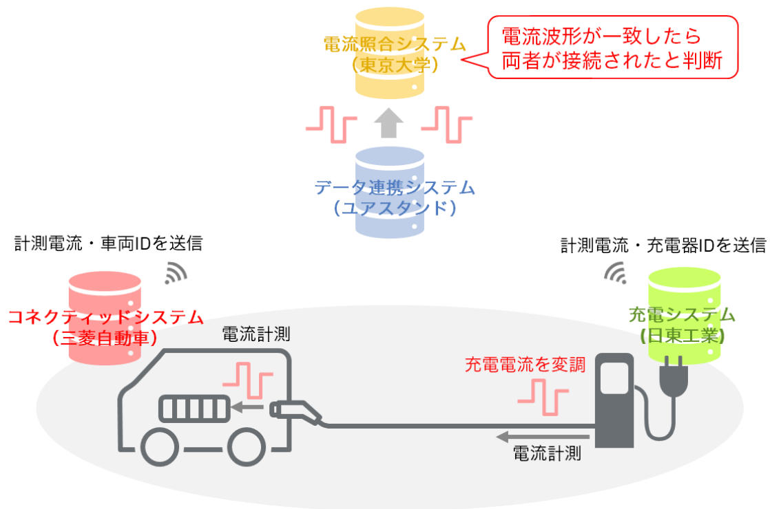
今般の実験システムの基本構成（充電器-EVを2組用意）
