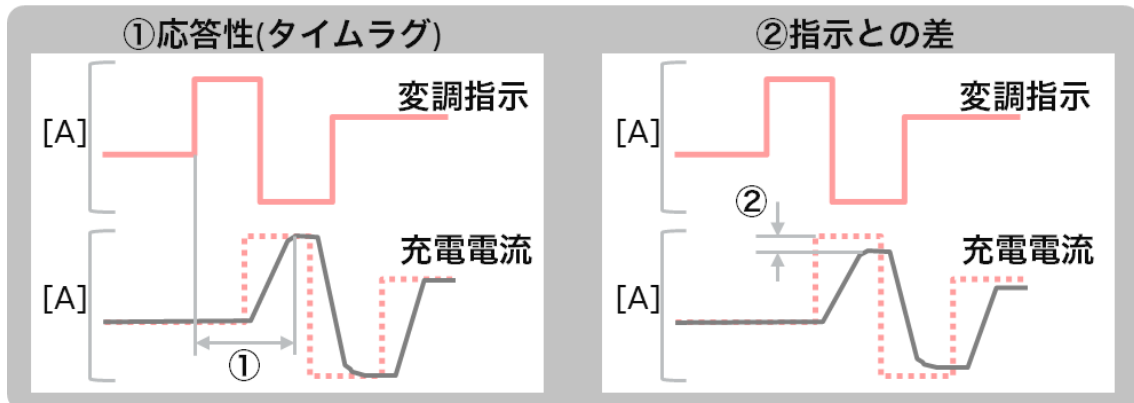
三菱自動車 軽商用EV『ミニキャブEV』の電流応答特性
