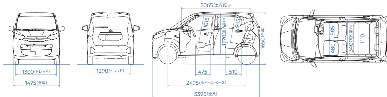
外観4面図 (G 2WD) 単位:mm
